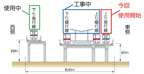
△駅部横断面図（完成イメージ）
