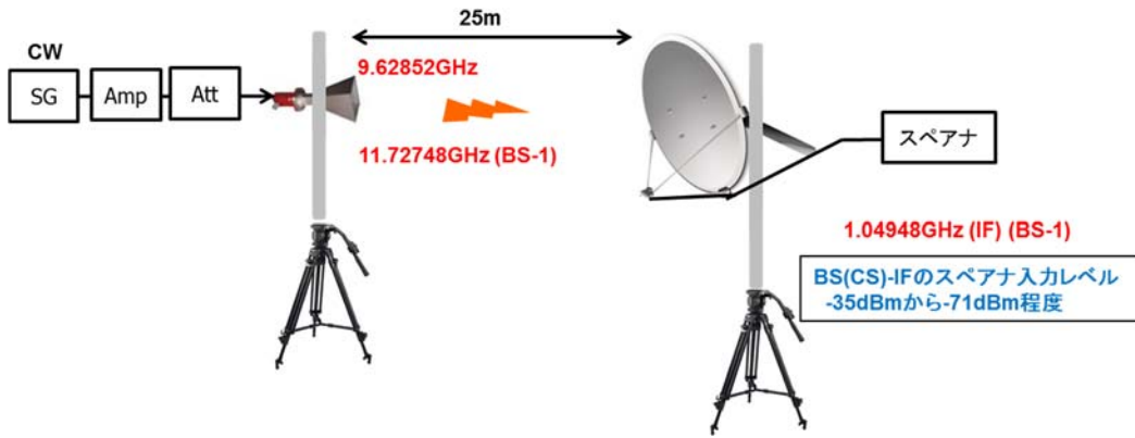
図 5 アンテナ放射パターン測定
