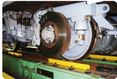
輪重測定
