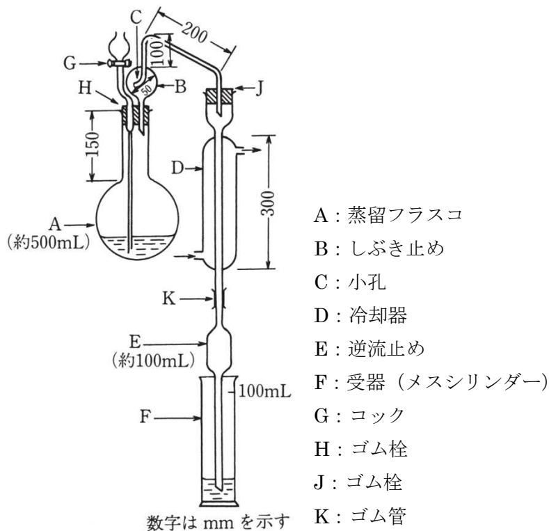
図 1 蒸留装置
