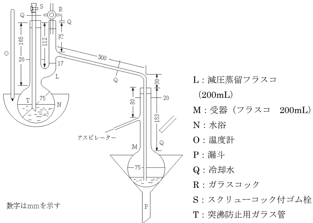
図2 減圧蒸留装置
