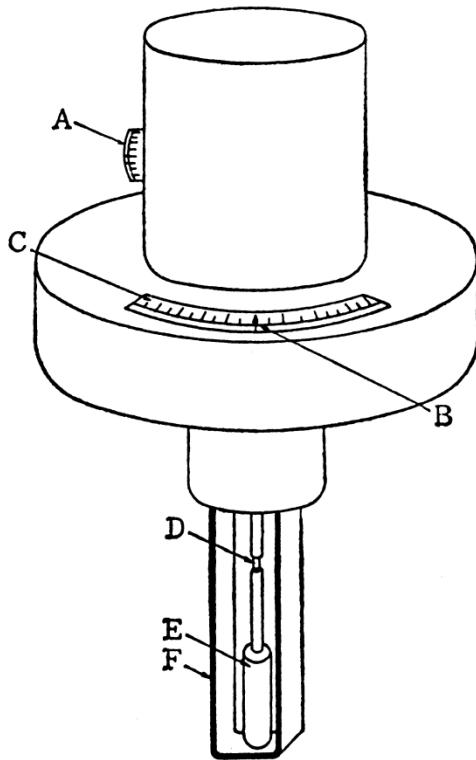
図2 回転粘度計
