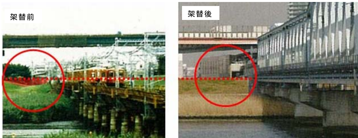
写真 4-19 京成押上線の架け替え
