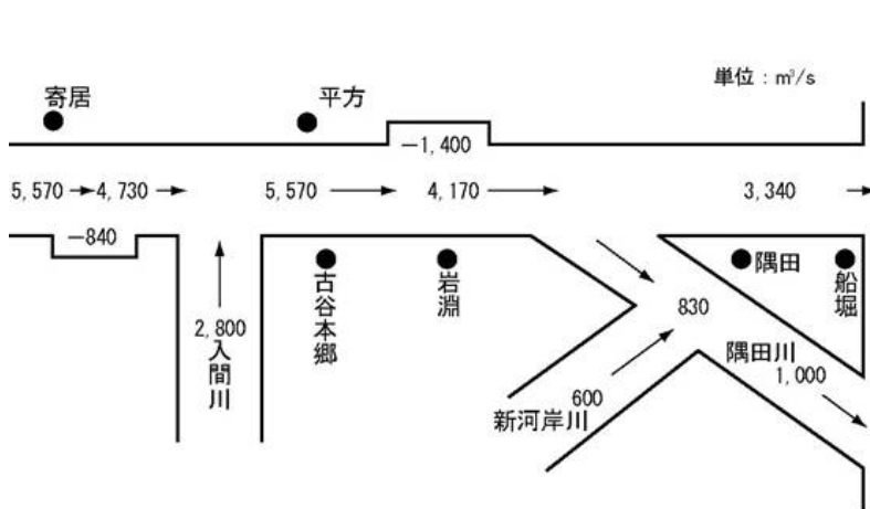
図 4-13 荒川計画高水流量配分図 流量は大正 7 年と同じ
