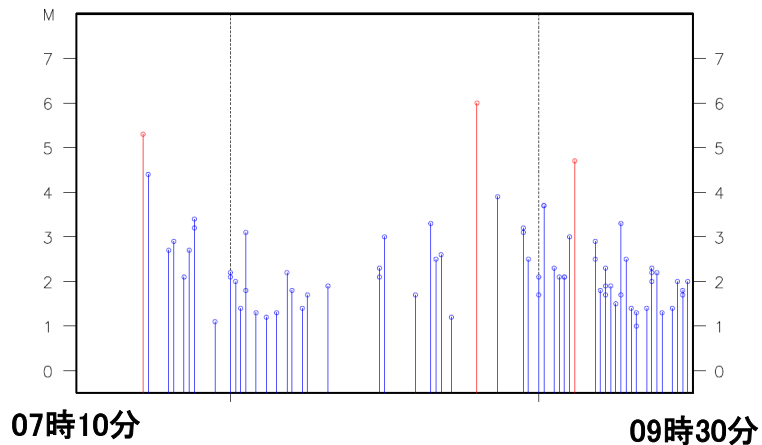
横軸は時間、縦軸はマグニチュード。縦棒のついた丸は地震発生時刻とマグニチュードの大きさを表す。
