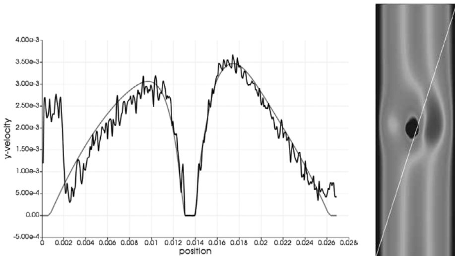
Abb. 2: Vergleich des Geschwindigkeitsprofils entlang einer Linie der Ebene (weiße Linie in der rechten Abbildung). Die experimentellen Daten werden als helle Linie dargestellt und die Simulationsergebnisse als dunkle Linie. Hier zeigt sich eine deutliche Reduzierung des Messrauschens.
