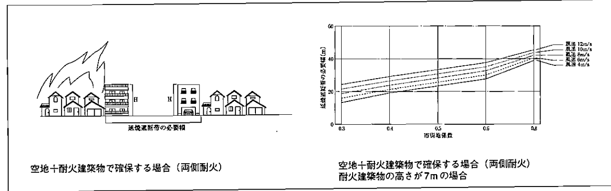
図7 延焼遮断帯の設計法(出典:ぎょうせい「都市防火実務ハンドブック」1997.9)
