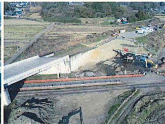
③ 跨道橋下部工事
