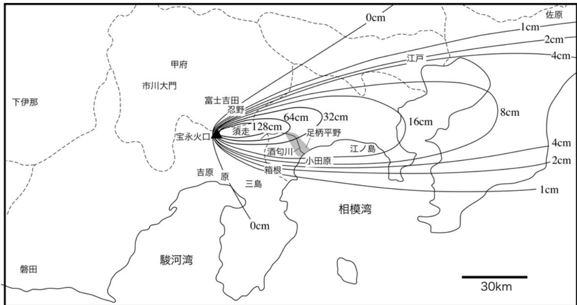
図 1-1 宝永噴火に関連する主な地名を示した地図
