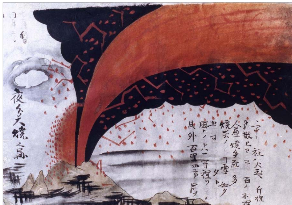
図 2-1 「浅間山夜分大焼之図」 (美齋津洋夫氏蔵)
