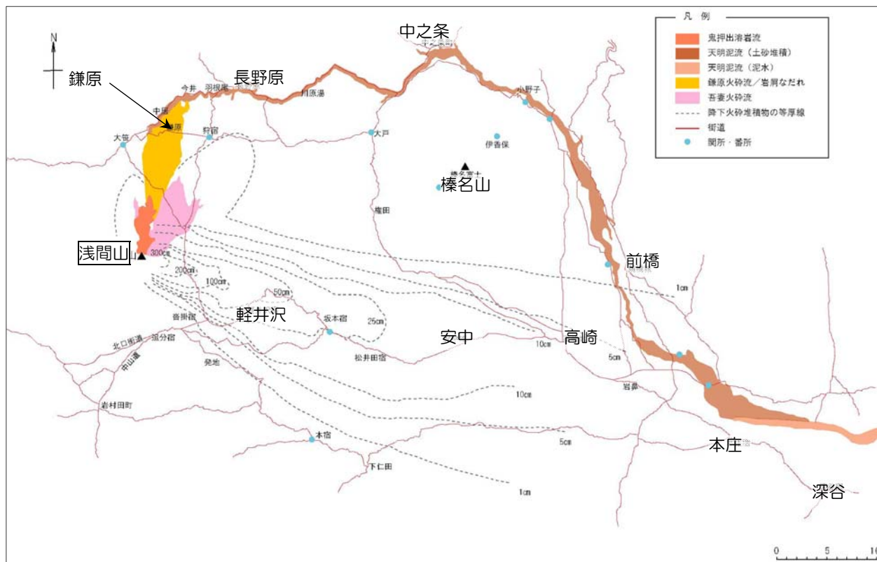
図 2-5 軽石・火山灰の降下・堆積分布
