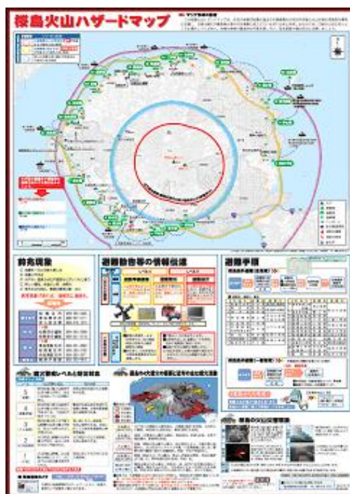
図 4-9 桜島火山ハザードマップ
