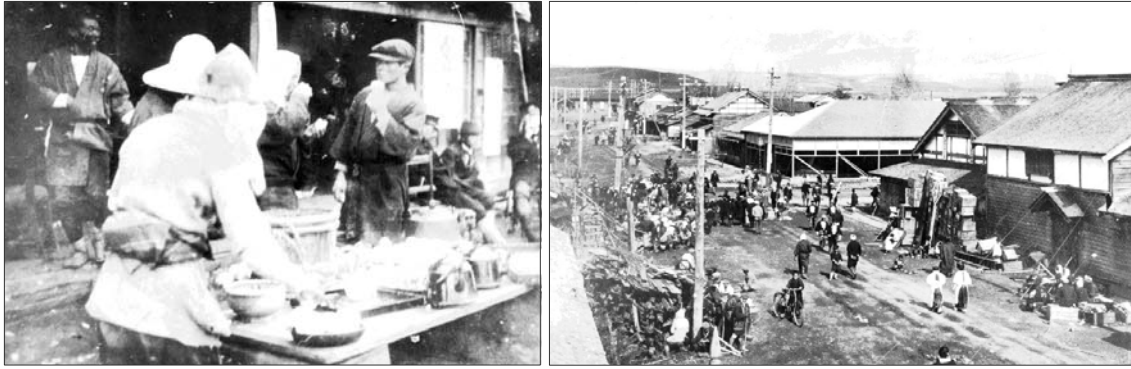
写真 5-4 (左) 救援本部前での炊き出し、(右) 救援に集まった地元上富良野の人々 (出典：写真 5-3 に同じ)
