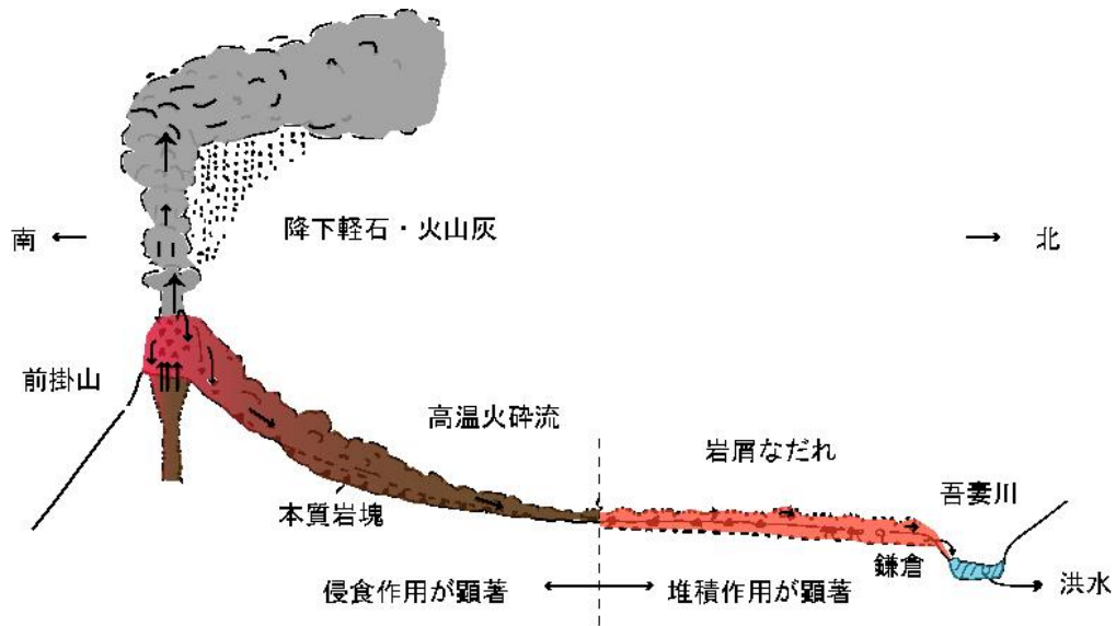
図 2-6 鎌原火砕流／岩屑なだれのモデル
