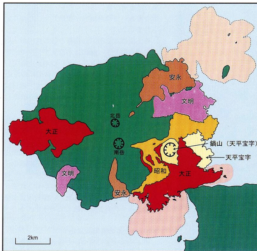
図 4-1 歴史時代の溶岩流
