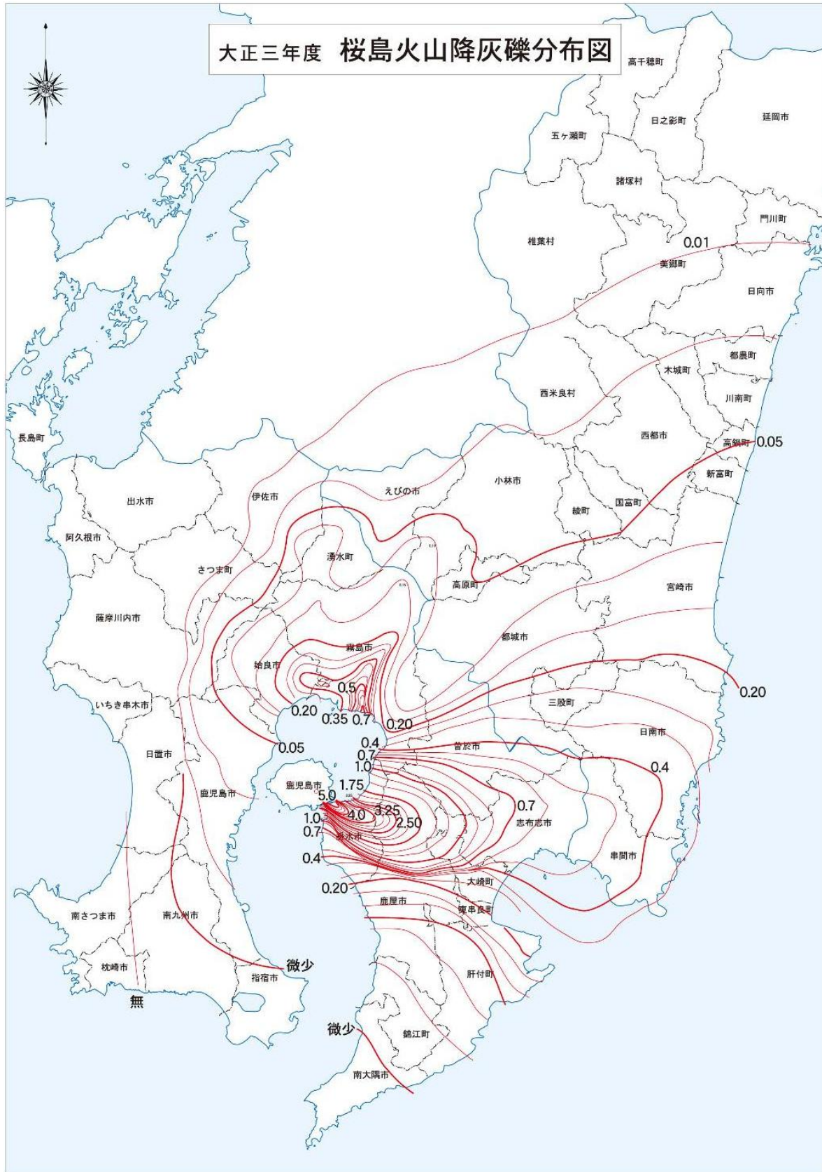
図 4-3 火山降灰礫分布図 (単位: 尺)
