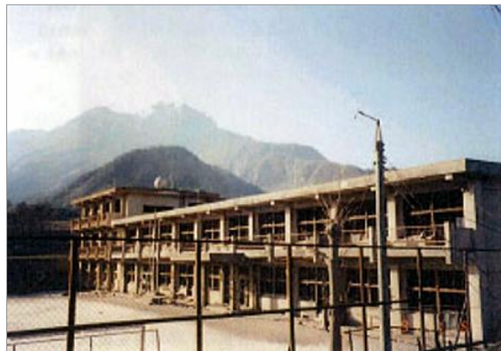
写真 6-3 1991(平成3)年9月15日の火砕流で 焼失した深江町立大野木場小学校
