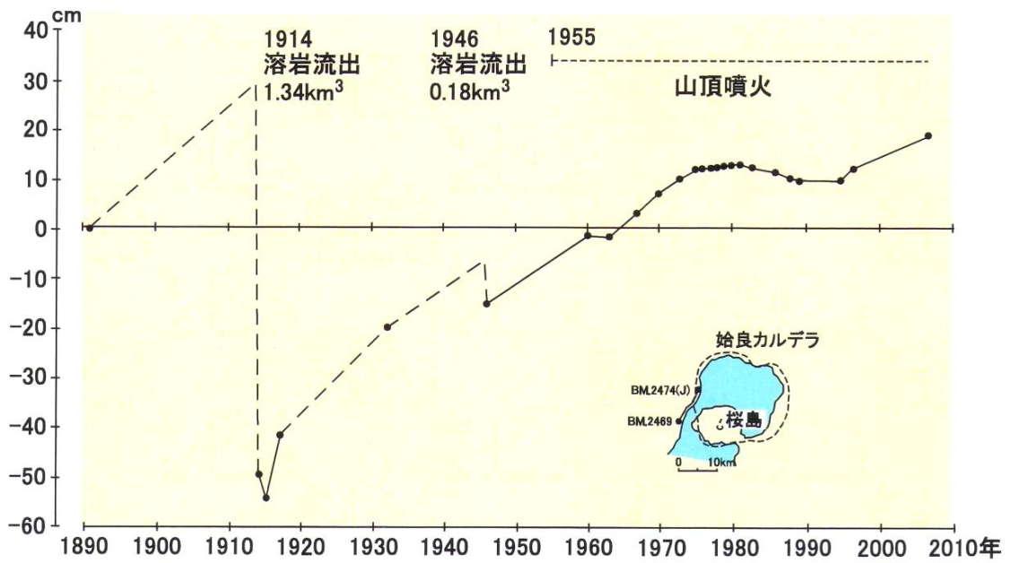
図 4-10 始良カルデラの地盤の昇降 (京都大学防災研究所他 (1987 年) を改訂)
