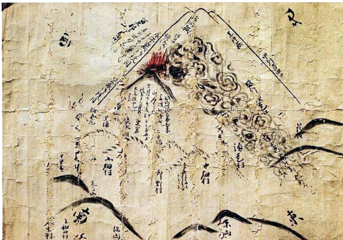
図 1-2 富士山宝永噴火之図 (静岡県御殿場市滝口文夫氏蔵)
