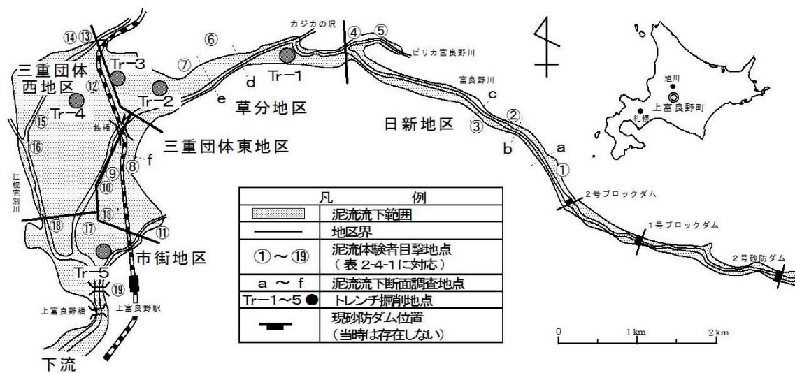
図 5-2 大正泥流体験者の目撃地点
