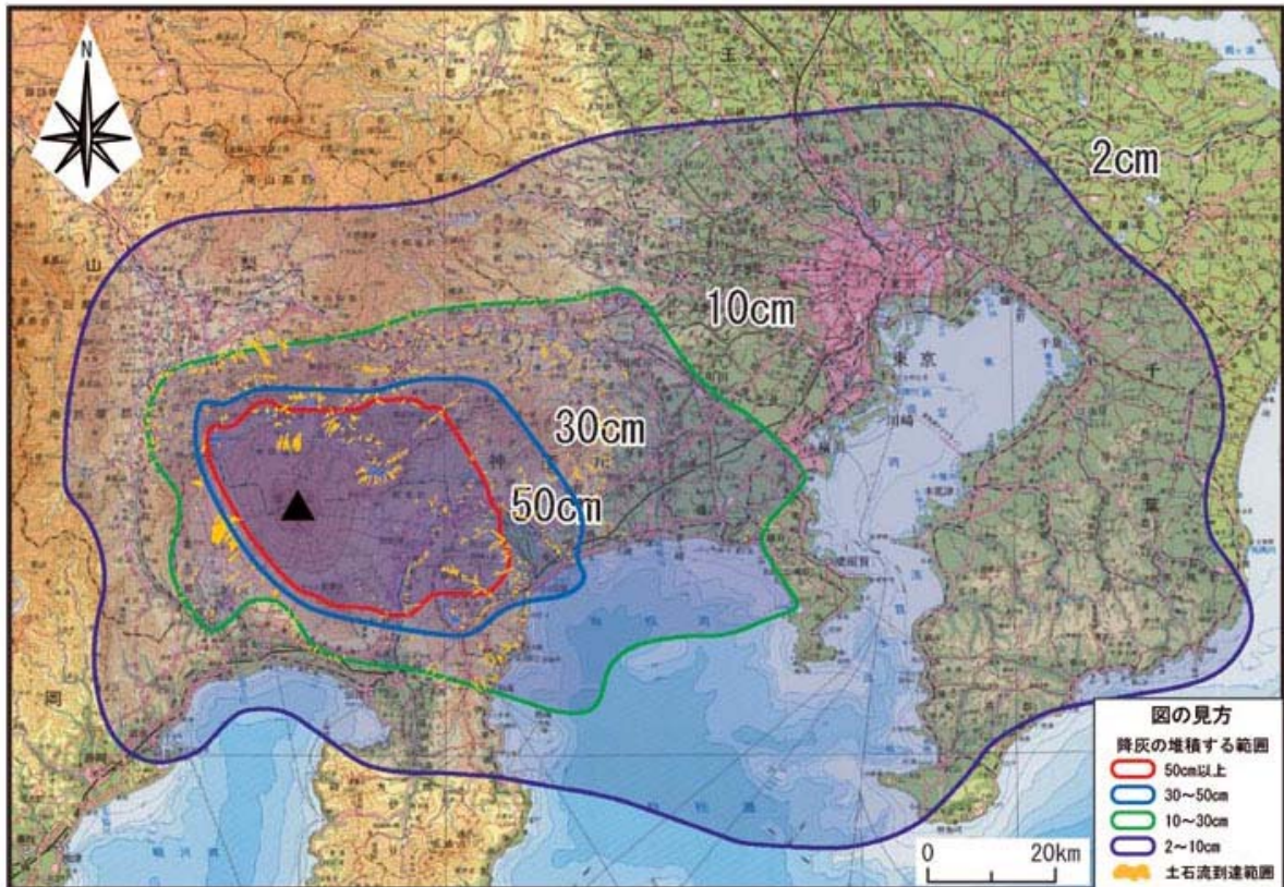
図 1-4 宝永噴火規模の噴火を想定した場合の降灰厚さと土石流の発生地点を予測したハザードマップ（『富士山ハザードマップ検討委員会報告書』平成 16 年 6 月より）
