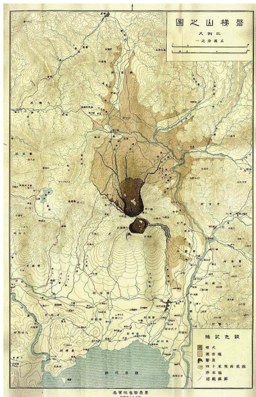
図3-2 噴火後の噴出物分布図 (農商務省地質局調査報告書(1889年) 掲載図。国立科学博物館蔵)
