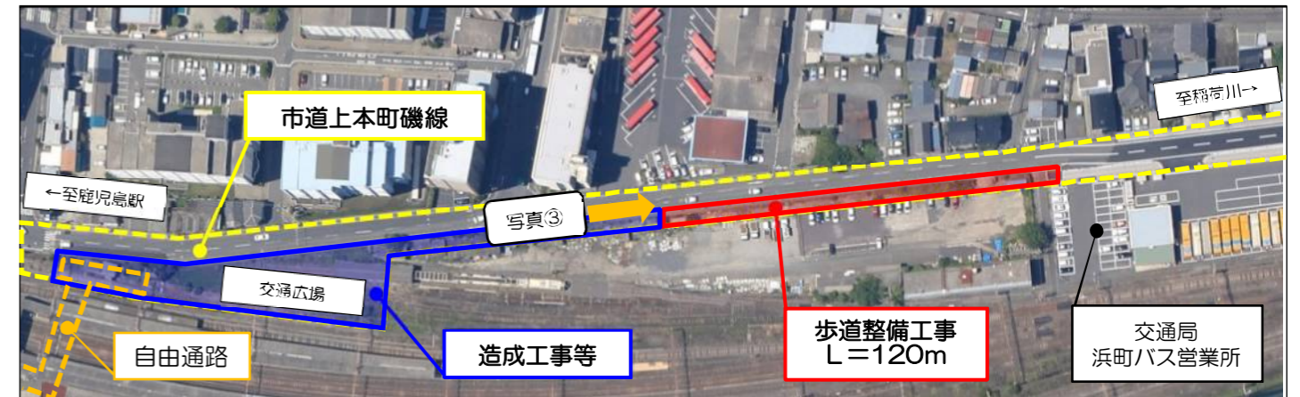
〈施工位置図〉
