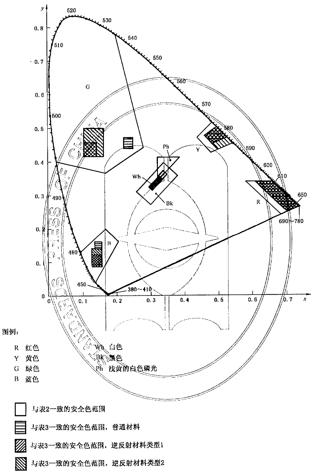
图 1 安全色和对比色的色品区域
