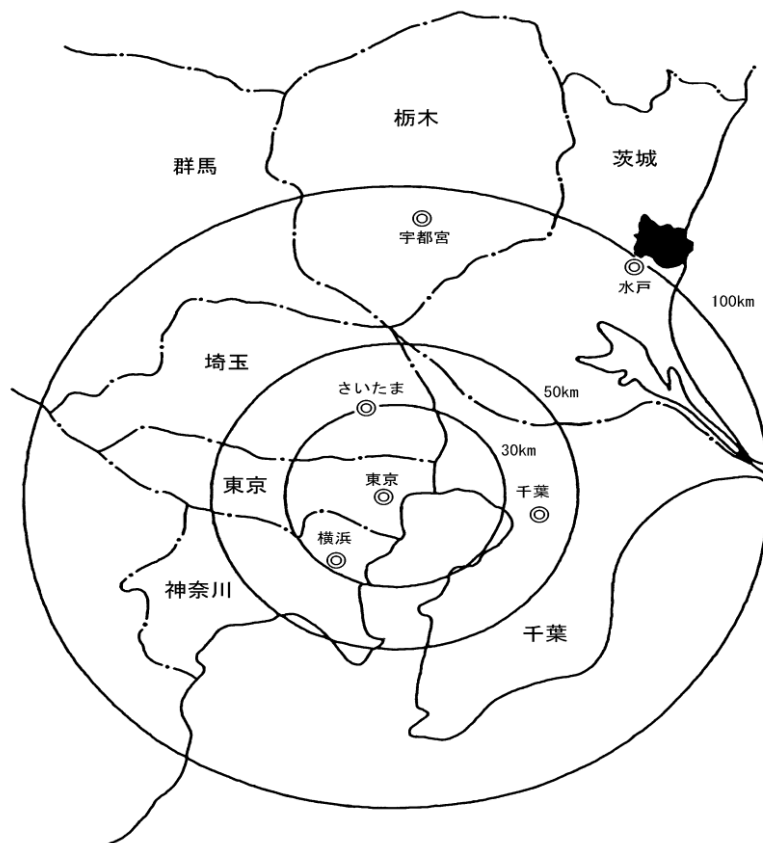
ひたちなか市位置図
