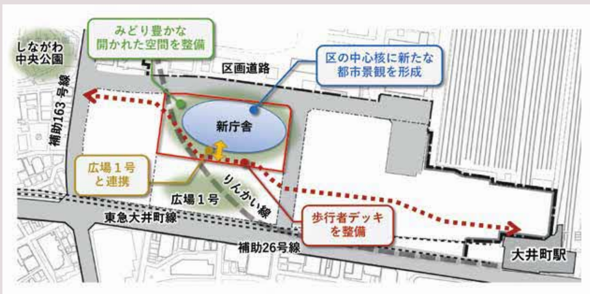
新庁舎の建物配置計画
