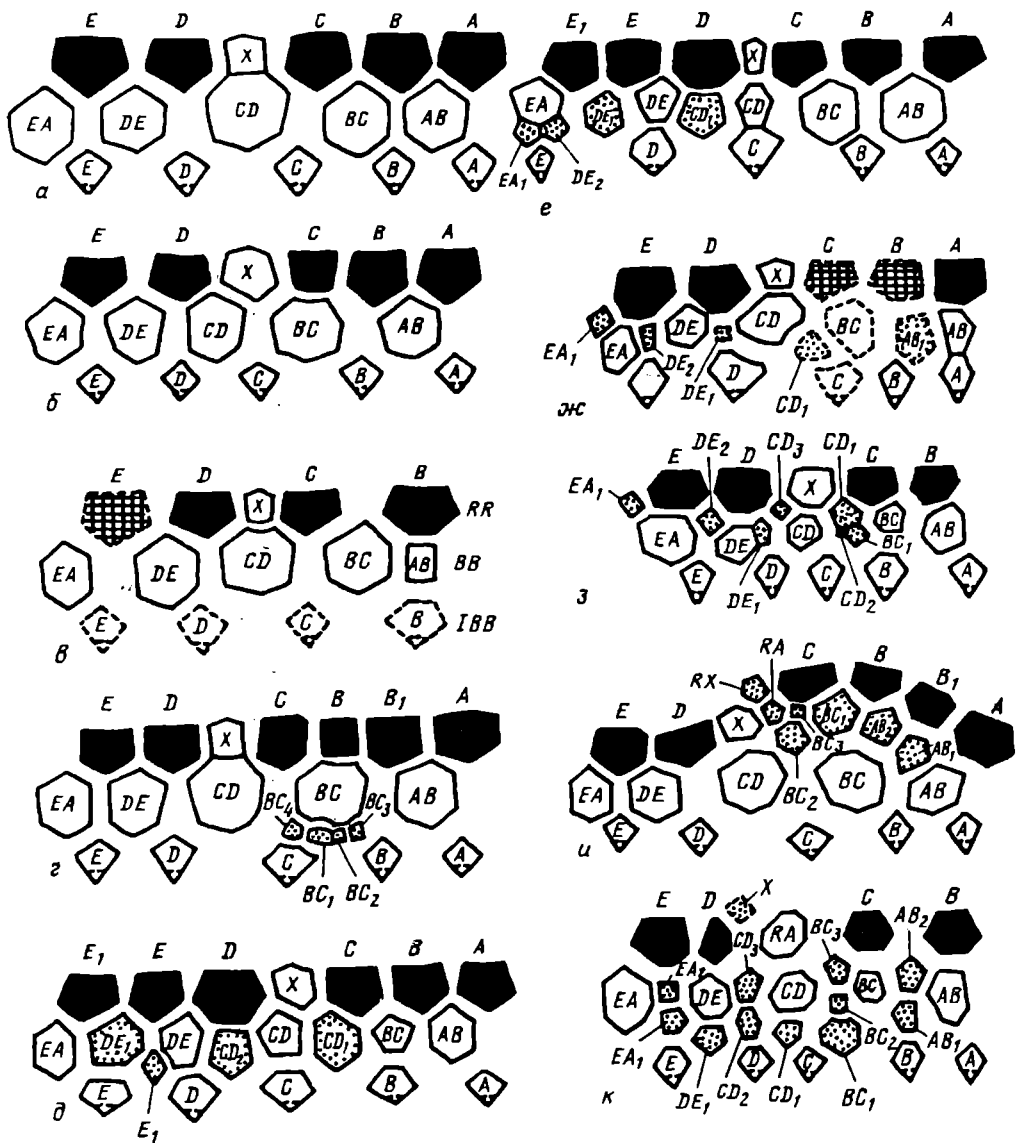
Рис. 2. Belashovicrinus gjelensis Arendt et Zubarev, sp. nov.; а — голотип ПИН, № 1641Б/109; б — к — aberrantные экз.: б — экз. № 1641Б/26; в — экз. № 1641Б/42; г — экз. № 1641Б/40; д — экз. № 1641Б/21; е — экз. № 1641Б/43; ж — экз. № 1641Б/41; з — экз. № 1641Б/44; и — экз. № 1641Б/24; к — экз. № 1641Б/110; условные обозначения см. на рис. 1
