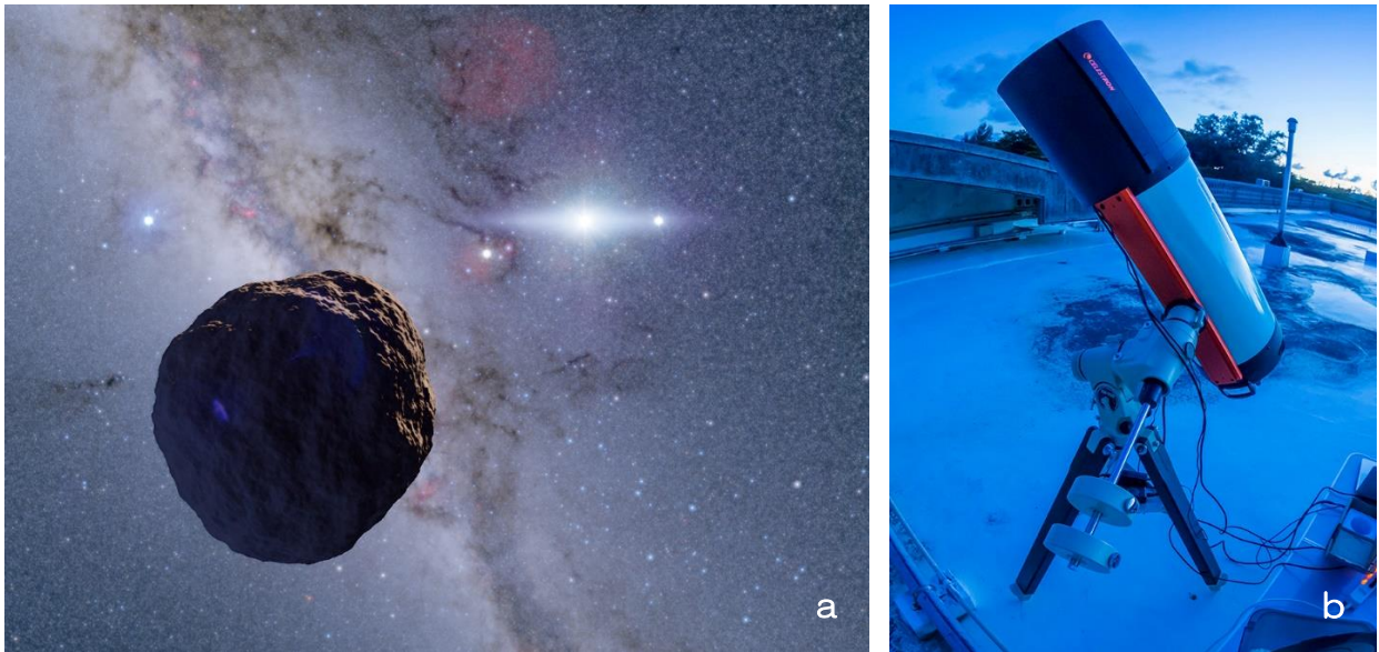
[図1] (a) 本研究によって史上初めて発見された、微惑星の生き残りとして推定される半径約 1.3km の小型カイパーベルト天体の想像図。(b) 巨大望遠鏡でも直接観測不可能な小型カイパーベルト天体を見つけた宮古島の口径 28cm 小型望遠鏡 (OASES 観測システム)
