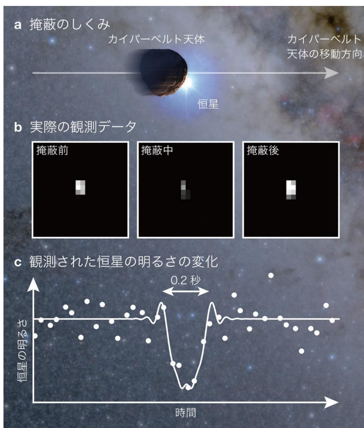
【図 3】「遮蔽」のしくみ (a) と今回の研究で発見された遮蔽のようす (b および c)
