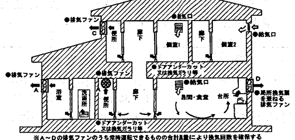
第三種換気 (ダクトを用いない方式、局所換気ファンと各室給気口の組み合わせ)
