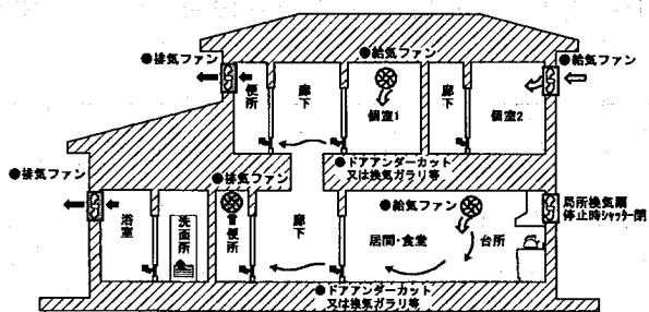
第一種換気 (ダクトを用いない方式、局所換気ファンと各室給気ファンの組み合わせ)
