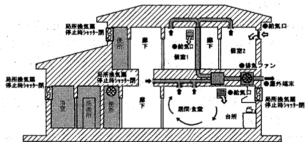
第三種換気 (ダクトを用いた方式)
