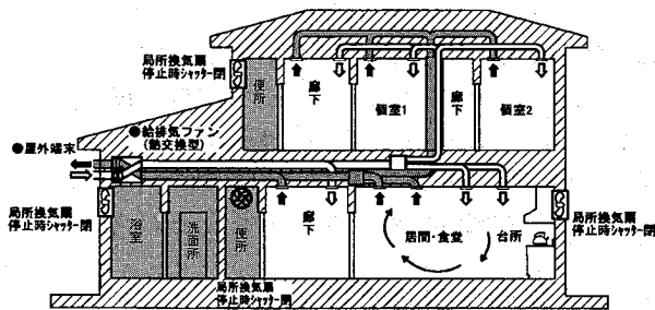
第一種換気 (ダクトを用いた方式)
