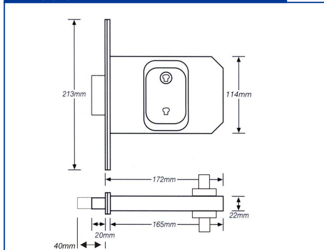
DIMENSIONS
